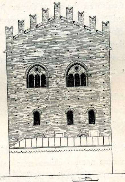
Tav. VIII. Disegno del ristauro.
